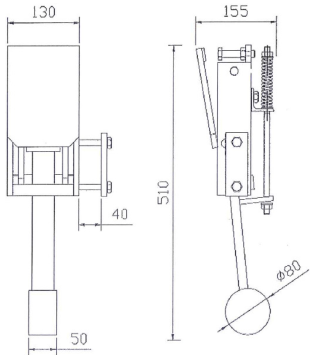
Marteau pour cloche < 100 kg (réf III224F)
